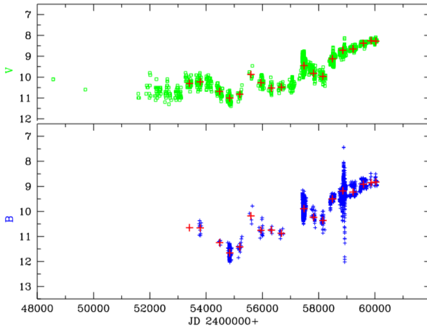
Фиг. 8. Криви на блясъка за периода от 1987 до 2023 на MWC560 по данни от AAVSO в В и V филтри. С червените плюсове са показани средните стойности за всеки наблюдателен сезон.
