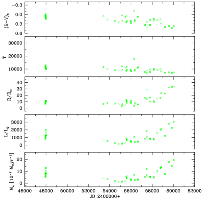
Фиг. 10. Еволюция на горещия компонент на MWC560. От горе на долу са представени (B - V)_0 с отчетена екстинкция, ефективна температура T[K] , ефективен радиус в слънчеви радиуси R/R_{\odot} , светимост в слънчеви светимости L/L_{\odot} , и темп на акреция M_a[10^{-7} M_{\odot} \text{yr}^{-1}] .
