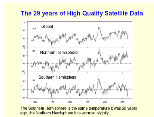
Фиг.2 Вляво: Изменение на среднопланетарната температура за периода 1850-2006 г (червената линия представя изгладените данни); вдясно: среднопланетарната температура по спътникови измервания (1978-2007 г)
