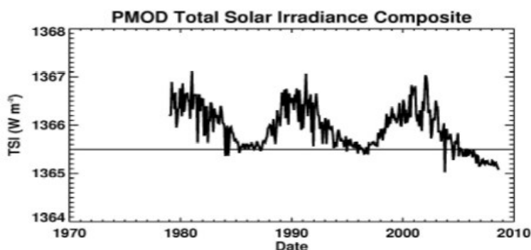
Фиг.6 11-годишна цикличност в изменението на общата слънчева светимост (индексът TSI) по спътникови данни. Последният слънчев минимум, който започна през 2005 година е свързан с по-дълбок минимум на TSI от предишните два.
