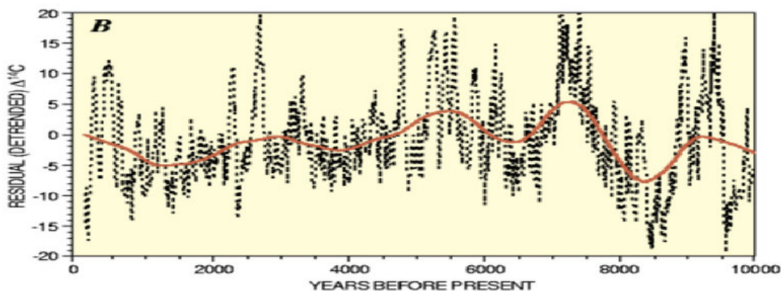
Фиг.8 2200-2400 годишния цикъл в съдържанието на радиовъглерод в годишните кръгове на дърветата. Хоризонталната ос предствя брой години назад в миналото.
